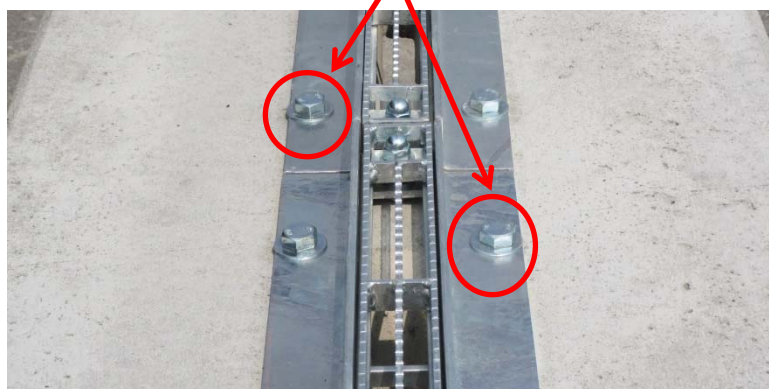
敷設後、座金+M16 ボルトを締め付ける
